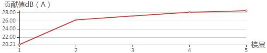
图 4-4 项目声源对洪桥街道黄山街居民点 5 贡献值
