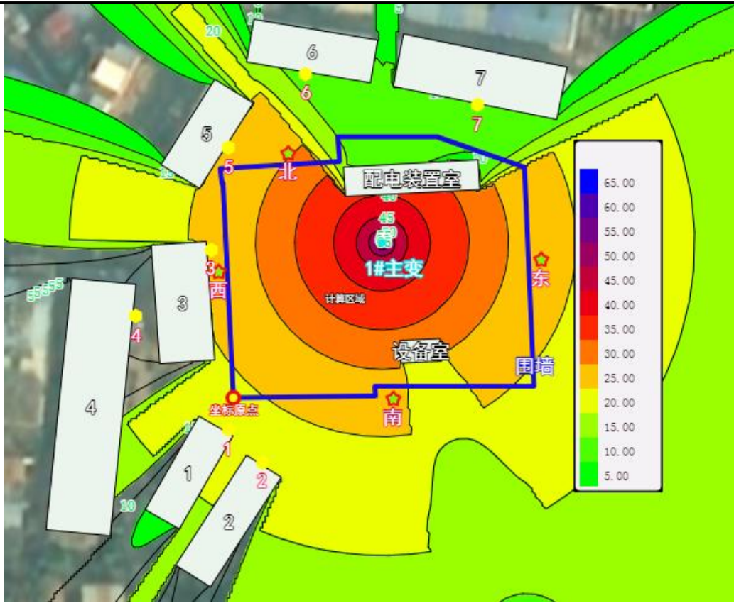
图 4-4 1#主变改造后噪声贡献值等值线图 (2.8m 高)
