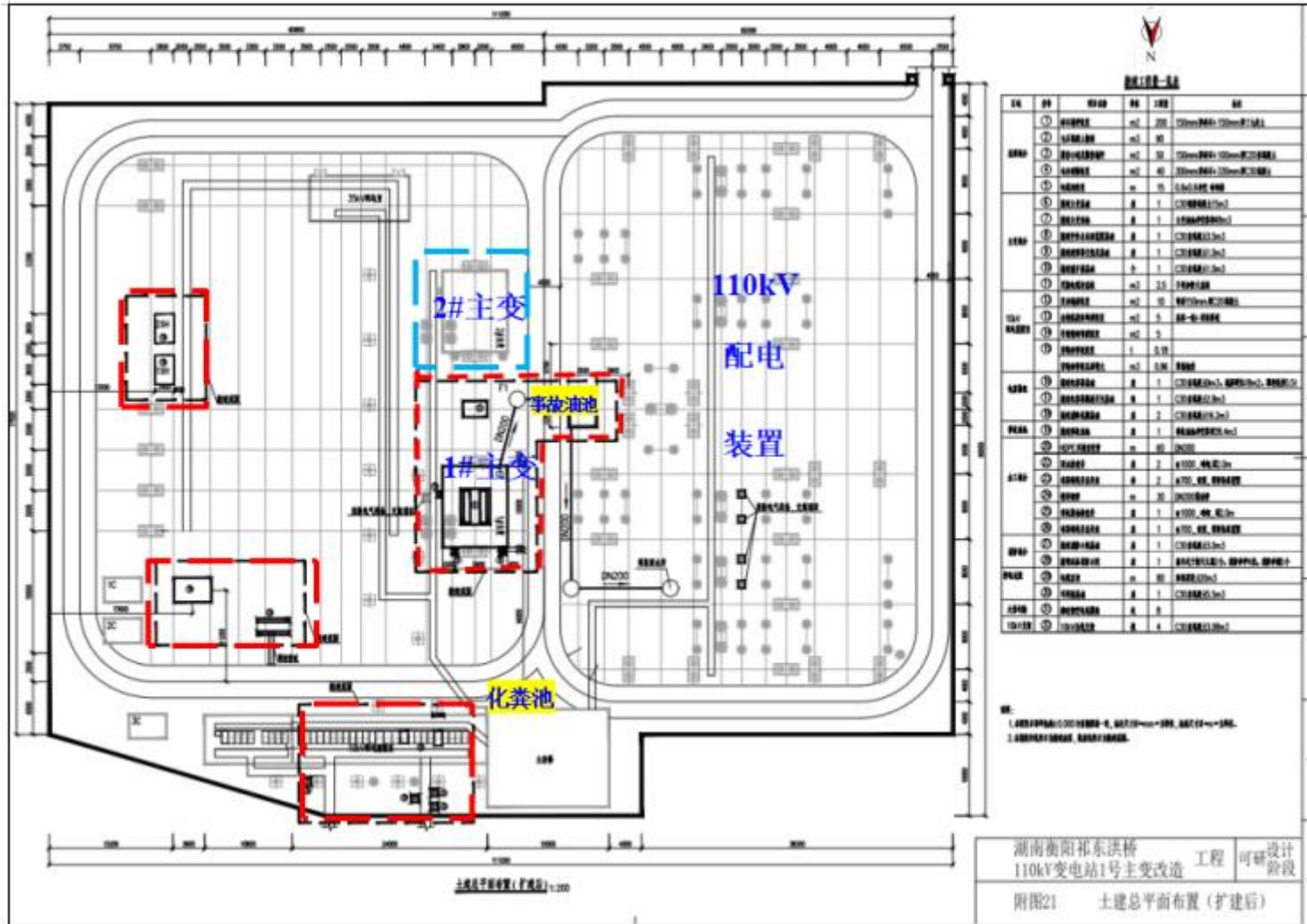
附图 3: 衡阳祁东洪桥 110kV 变电站改造后总平面布置示意图
