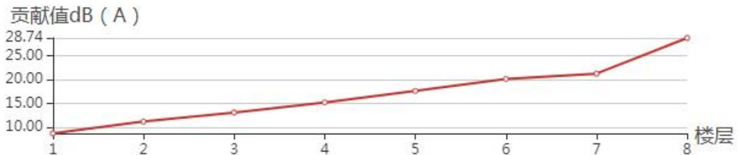
图 4-4 项目声源对洪桥街道黄山街居民点 7 贡献值
