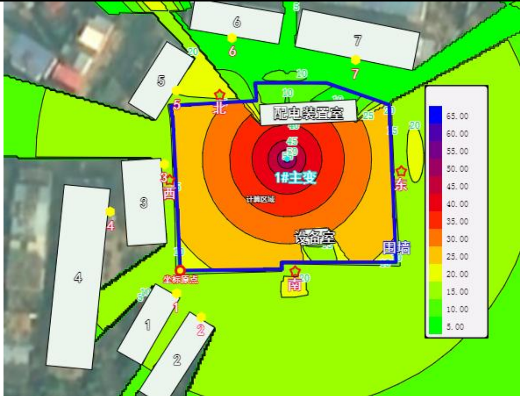
图 4-3 1#主变改造后噪声贡献值等值线图 (1.2m 高)
