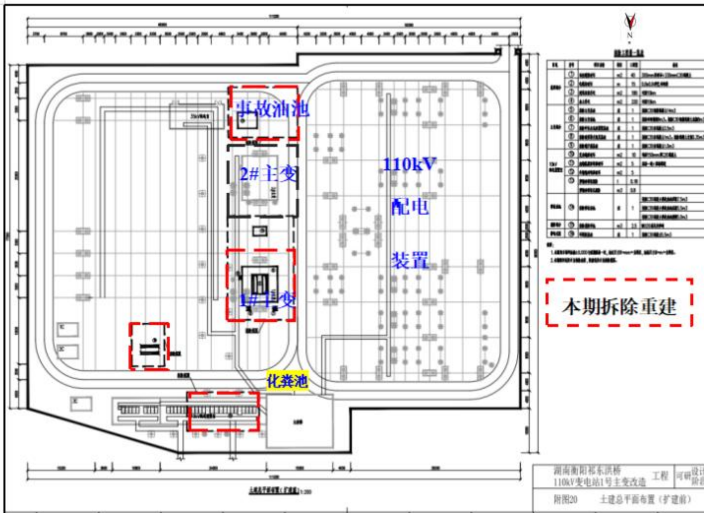
附图 2: 衡阳祁东洪桥 110kV 变电站现状总平面布置示意图
