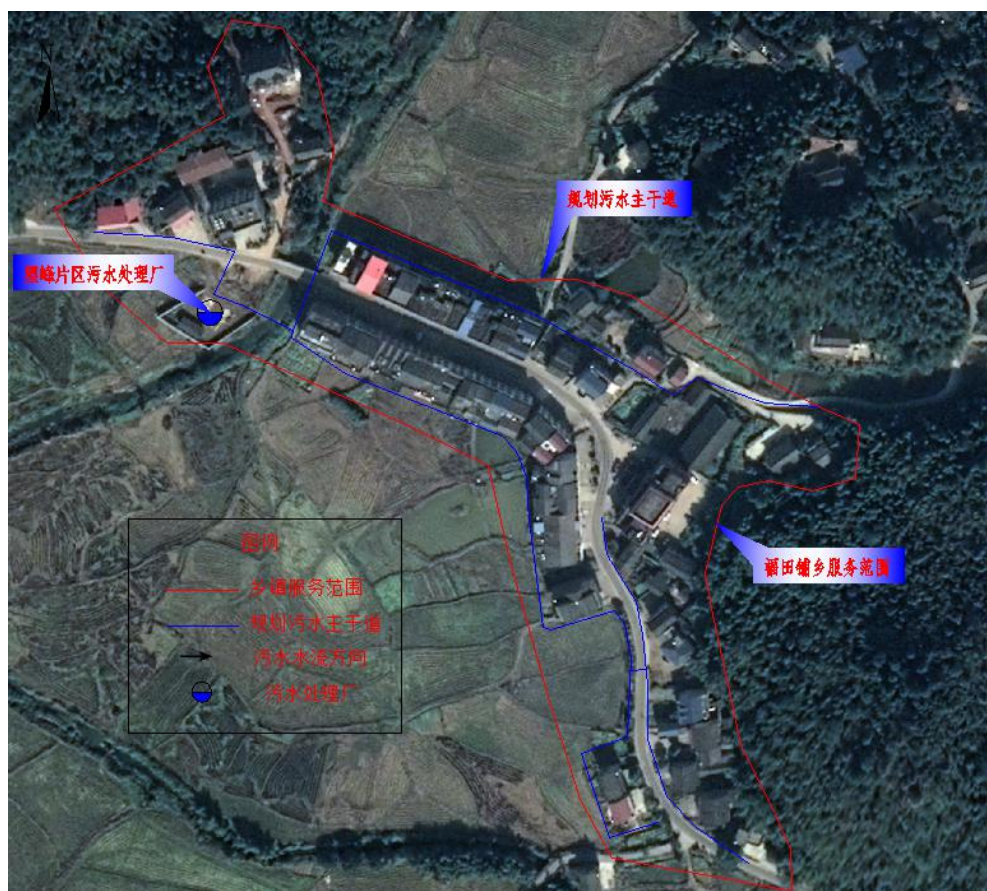
图 2.1-1 污水范围规划图
